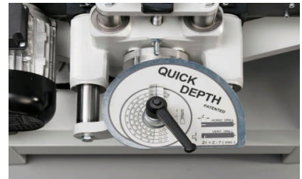
Quick depth Bohrtiefeneinstellsystem
