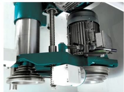
Fünf Drehzahlen mit Umlegen des Riemens
