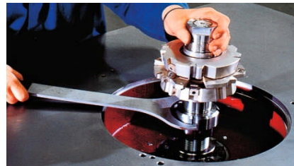
Auswechselbare Frässpindel
