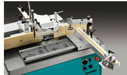
Einsatz mit Schlitztisch (Option)
