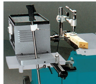
Dübelrastertrommel mit Arretierung am Handgriff
