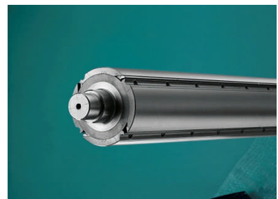
Monobloc Tersawelle (Option)
